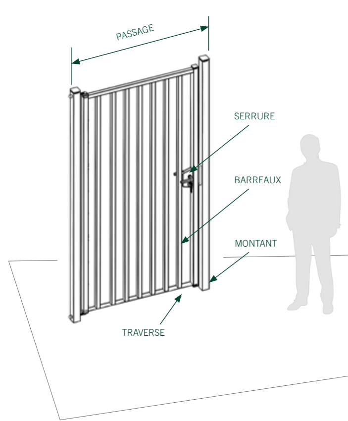
PORTAIL À UN SEUL VANTAUX Ouverture intérieure droite (standard)
