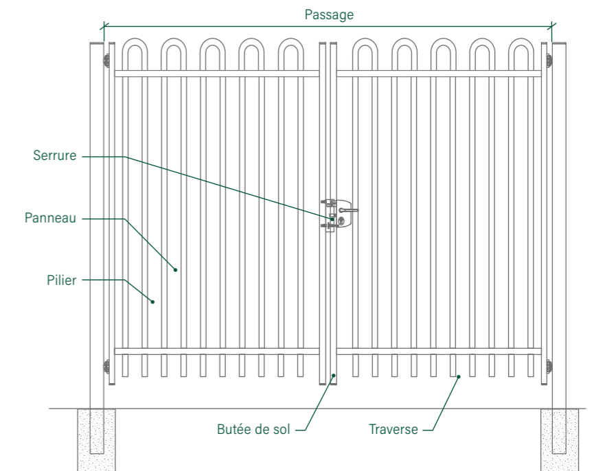
PORTAIL À DEUX VANTAUX Ouverture intérieure (standard)
