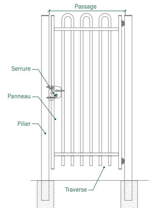
PORTAIL À UN SEUL VANTAUX Ouverture intérieure droite (standard)
